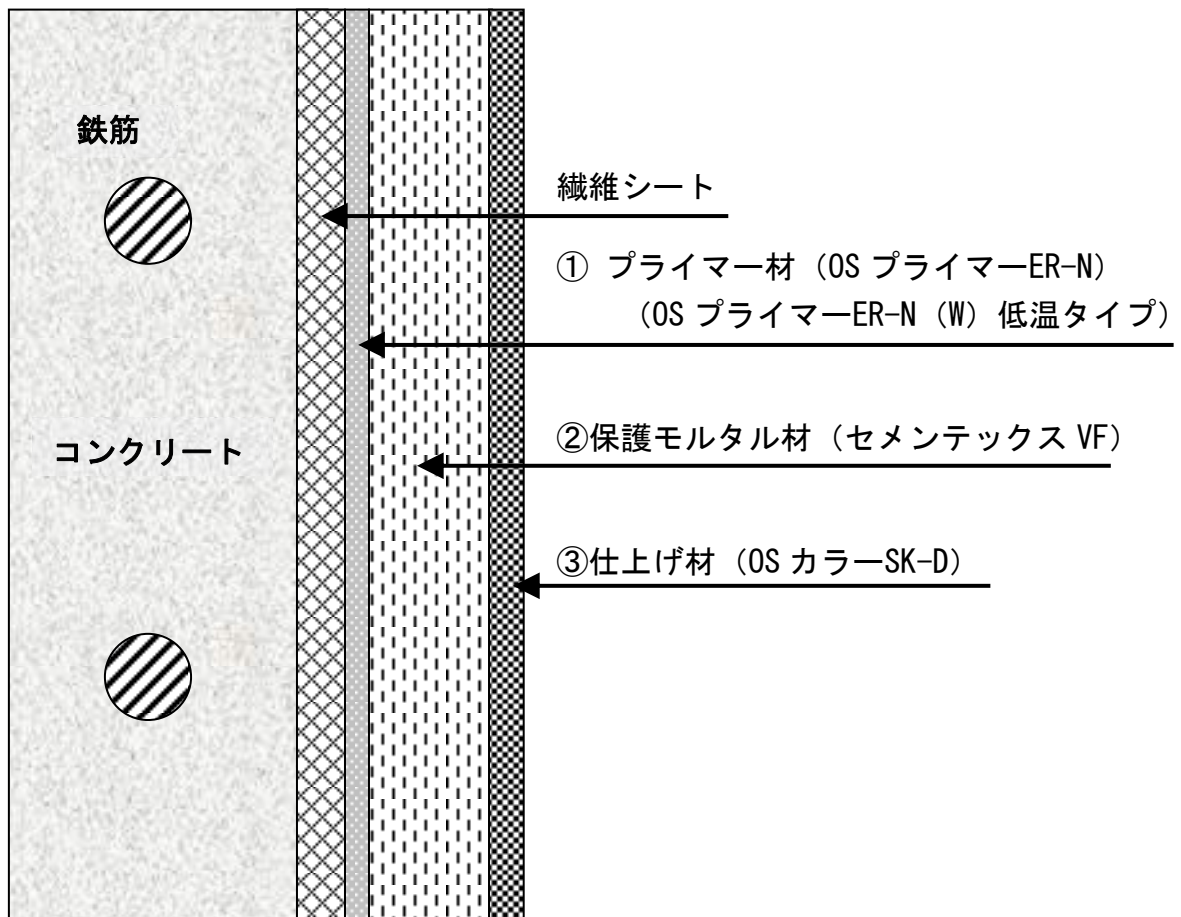
施工図
