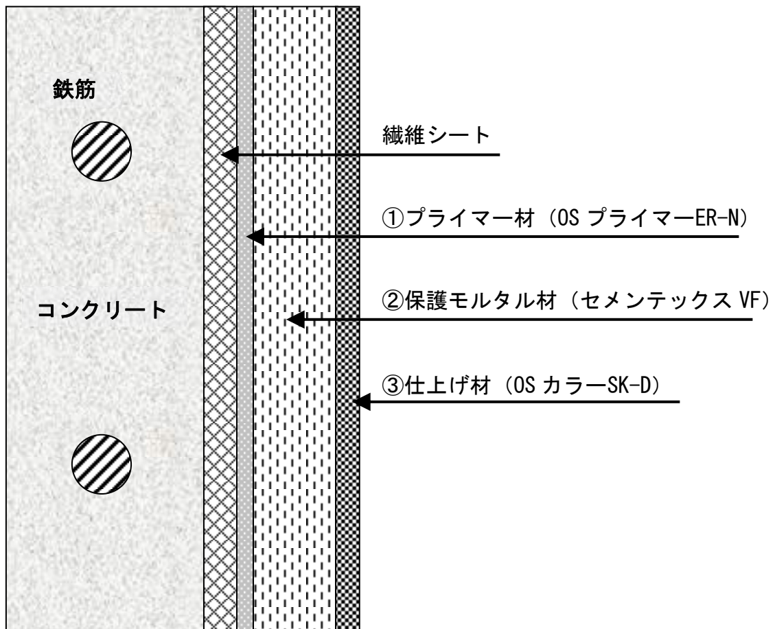
施工図
