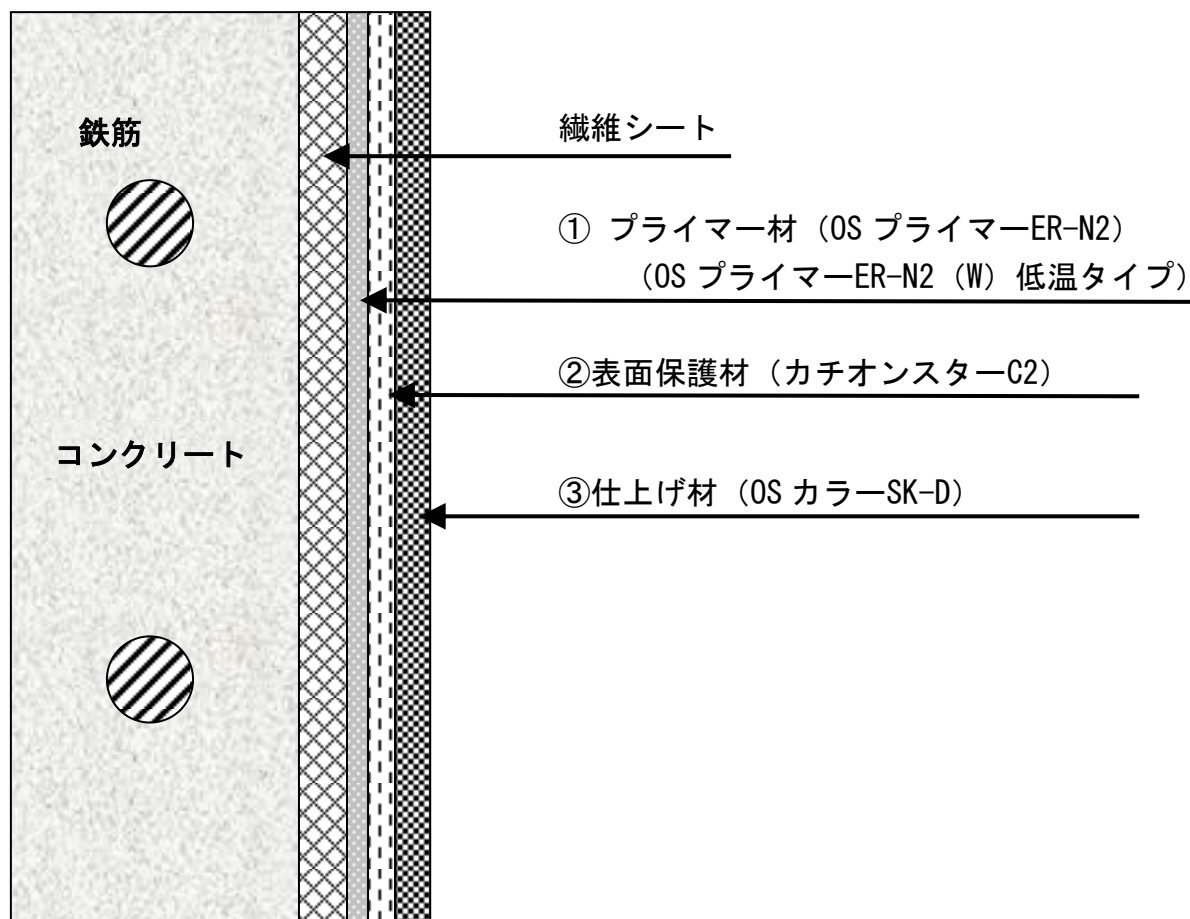
施工図
