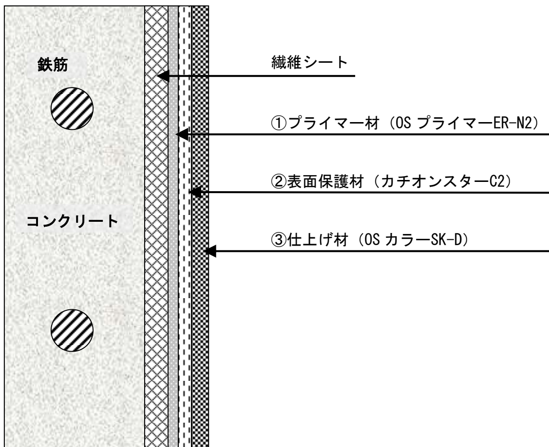
施工図
