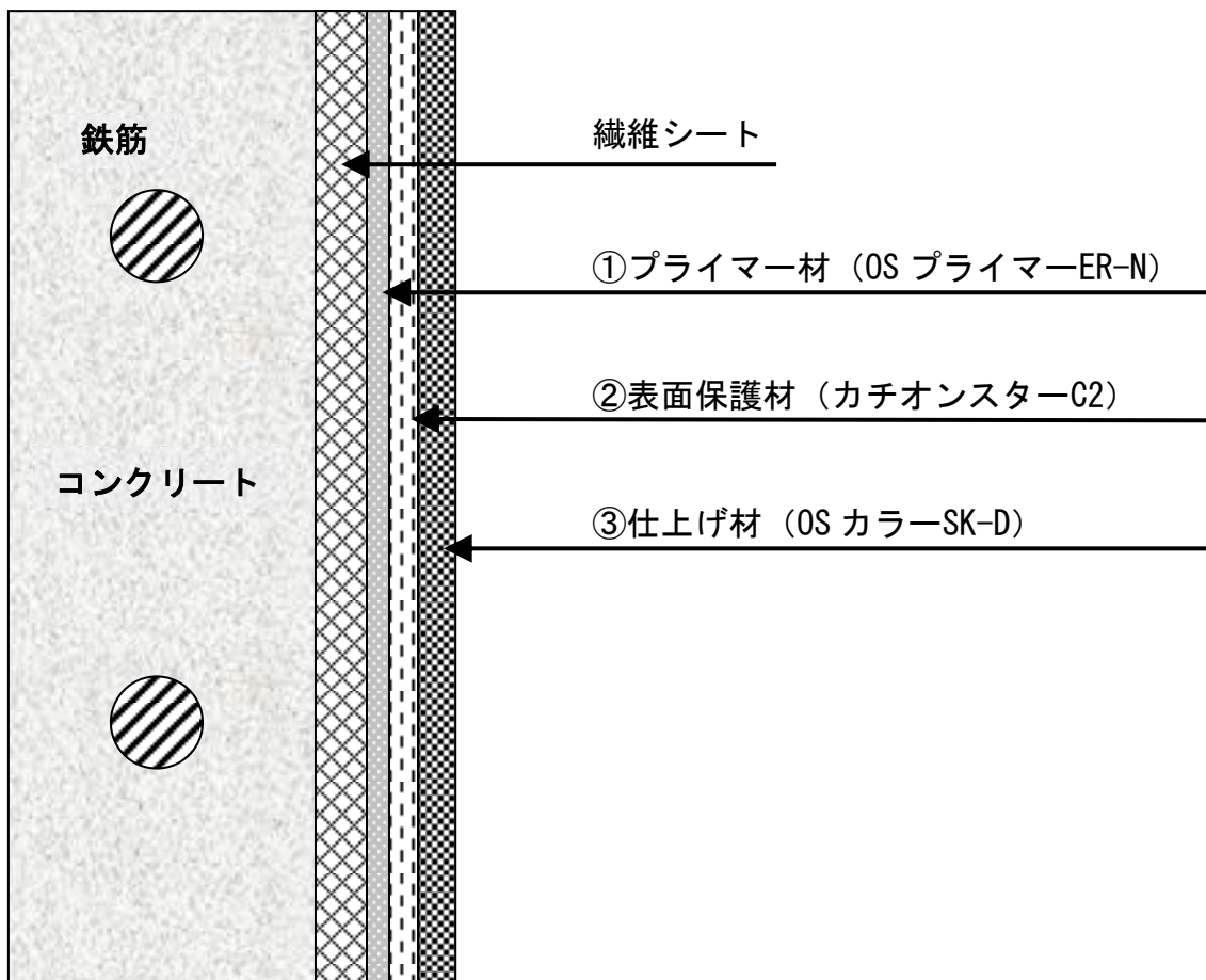
施工図
